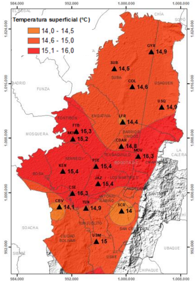
Figura 28. Mapa del promedio de temperatura superficial de las estaciones RMCAB con base en el método de interpolación de Kriging – enero 2022
