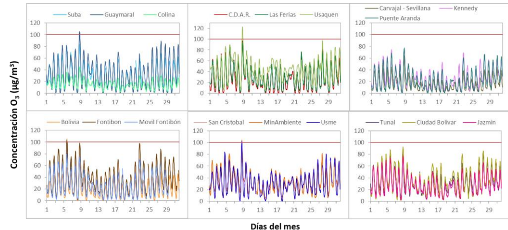
Figura 10. Concentraciones media móvil 8 horas de O 3 por estación de monitoreo - enero 2022
