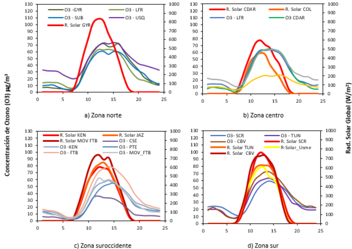
Figura 11. Comportamiento horario de las concentraciones de O 3 (µg/m 3 ) y su relación con la Radiación Solar entrante (W/m 2 ) – enero 2022. a) zona norte, b) zona centro, c) zona suroccidente y d) zona sur
