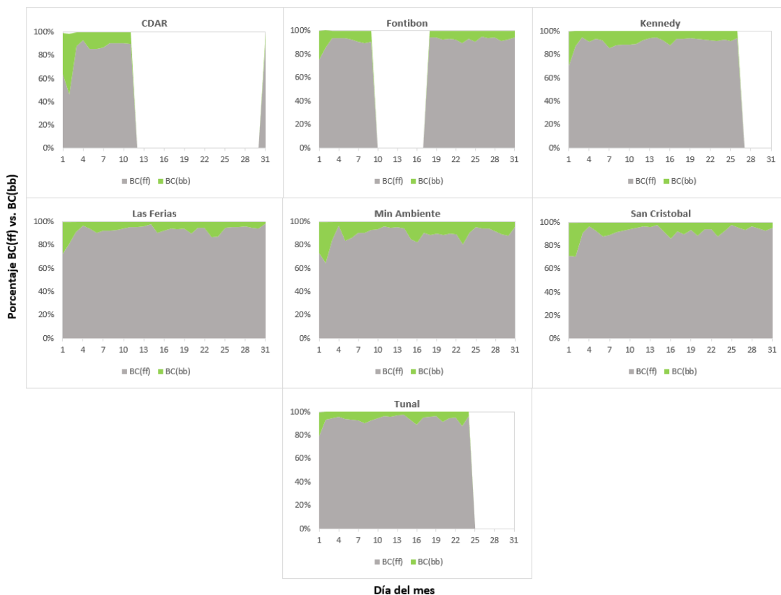
Figura 21. Serie temporal porcentaje de quema Black Carbon de combustibles fósiles BC(ff) vs. Black Carbon de quema de biomasa BC(bb) – enero 2022
