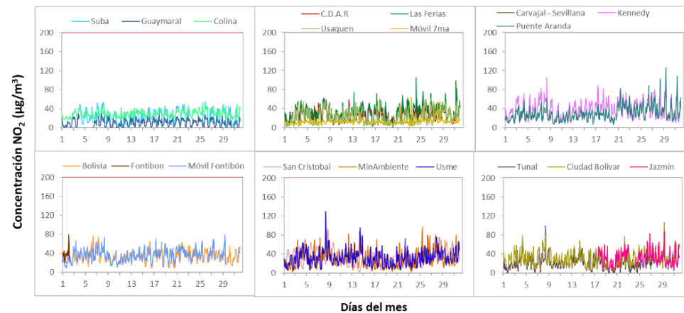
Figura 15. Concentraciones promedio mensuales de NO 2 por estación de monitoreo - enero 2022
