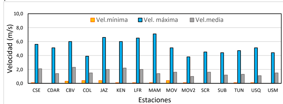
Figura 31. Velocidad del viento media, máxima y mínima absolutas por estación – enero 2022
