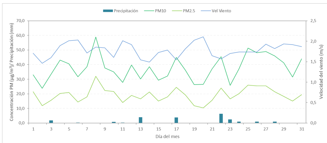
Figura 6. Promedio de concentración PM 10 y PM 2.5 , precipitación y velocidad del viento a nivel ciudad – enero 2022
