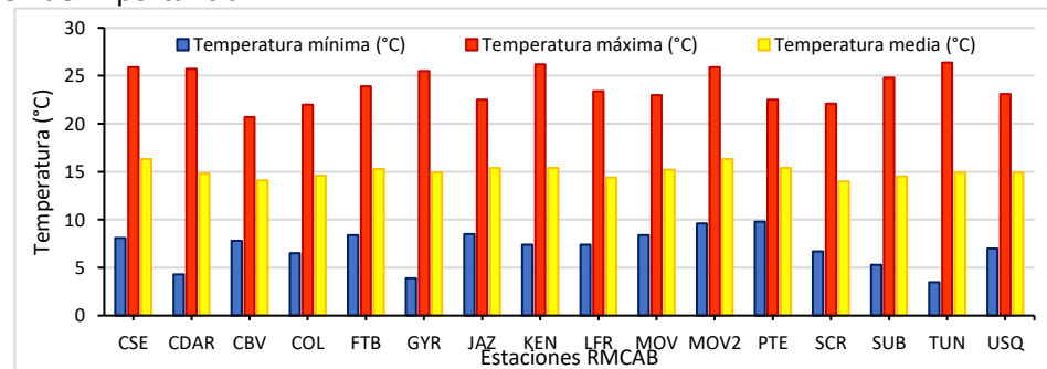
Figura 29. Temperaturas medias, máximas y mínimas absolutas por estación – enero 2022
