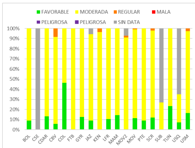
Figura 23. IBOCA para PM 2.5 por estación – enero 2022
