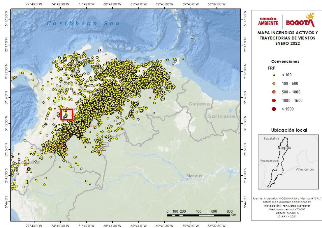
Figura 19. Distribución espacial de incendios activos identificados por el sensor MODIS en el mes de enero 2022
