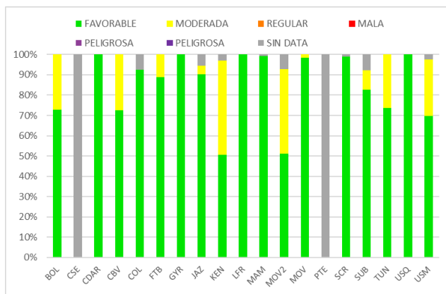
Figura 22. IBOCA para PM 10 por estación – enero 2022
