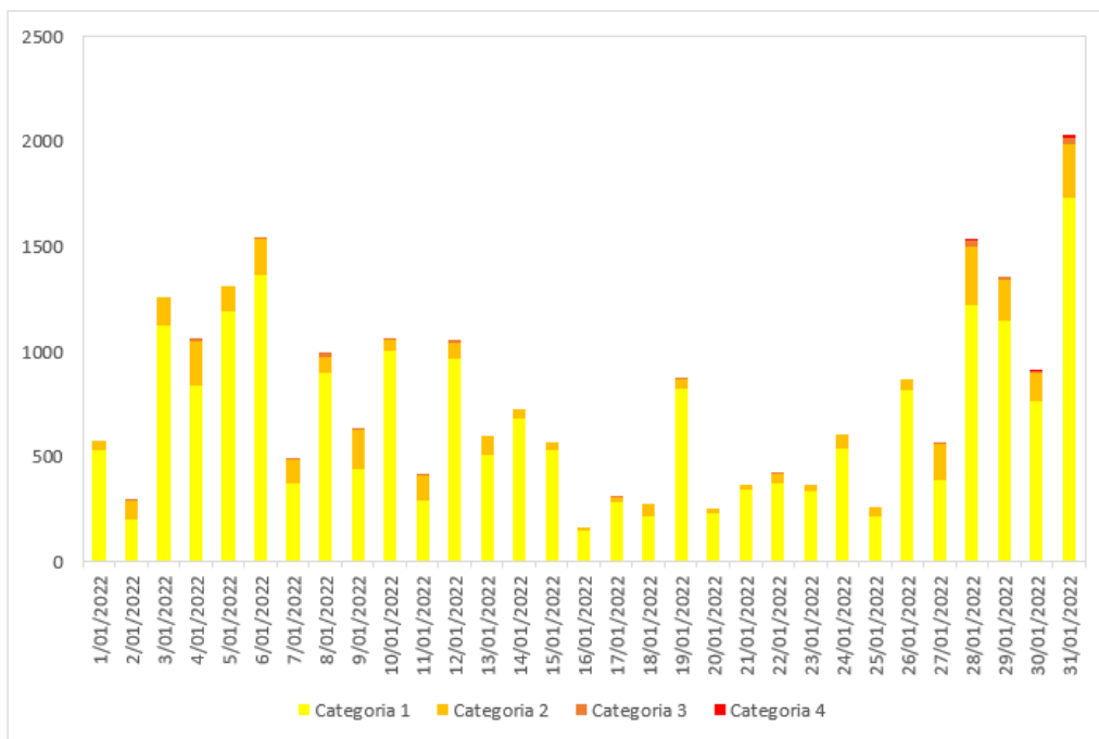
Figura 20. Número de eventos o puntos calientes identificados por el sensor MODIS en el mes de enero 2022
