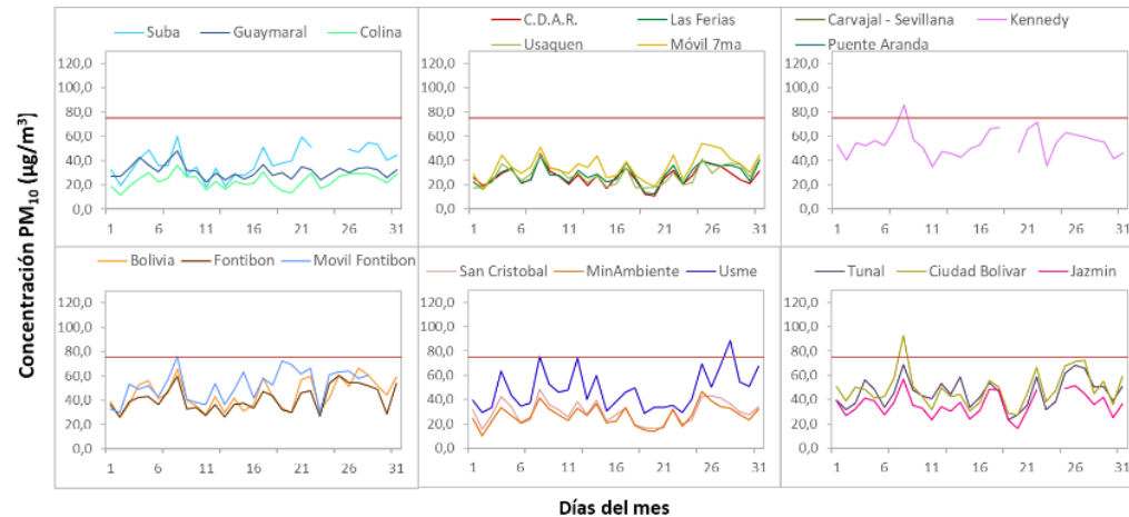
Figura 3. Concentraciones diarias PM 10 por estación de monitoreo – enero 2022
