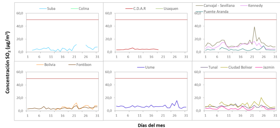
Figura 13. Concentraciones promedio mensuales de SO 2 por estación de monitoreo - enero 2022
