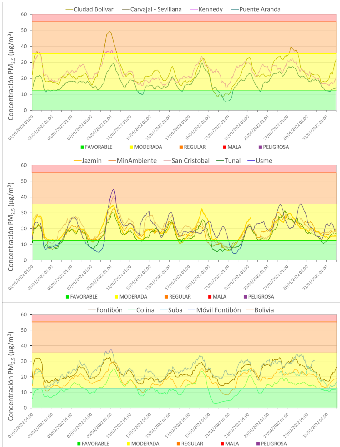
Figura 25. Concentraciones media móvil 24 h PM_{2.5} enero 2022
