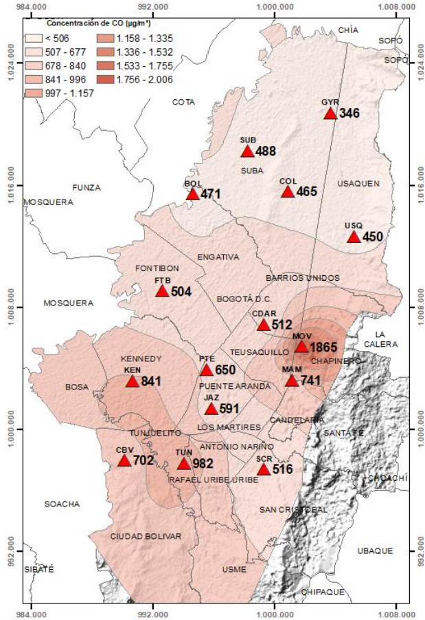
Figura 16. Distribución espacial concentraciones mensuales CO – enero 2022
