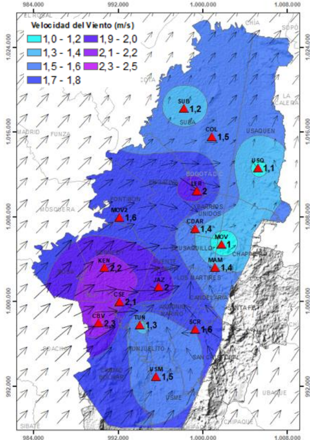
Figura 30. Velocidad promedio (Superficie en colores) y Dirección promedio (Vectores) del Viento con base en la interpolación de Kriging – enero 2022
